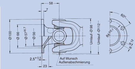
Beiderseits Flansch für größeren Beugungswinkel Endnummer: 0.110.XX5
