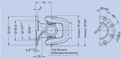
Beiderseits Flansch für größeren Beugungswinkel Endnummer: 0.113.XX5
