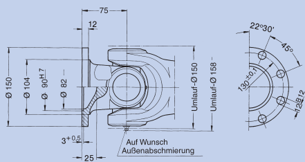
Normalfansch Endnummer: 0.158.XX0
