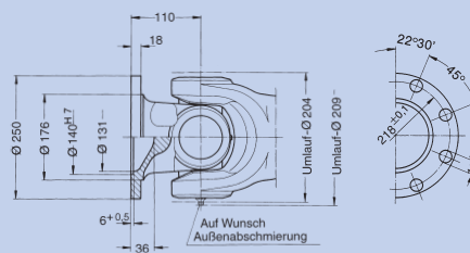
Größerer Flansch (Ø 250 mm) Endnummer: 0.122.XX1
