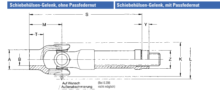
Passfedernut nach DIN 6885, Blatt 1
