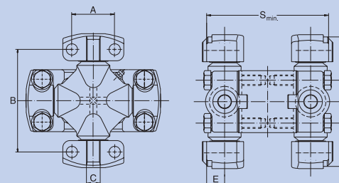
Bauform 300 Gelenk – doppelt Endnummer: 0.9XX.300
