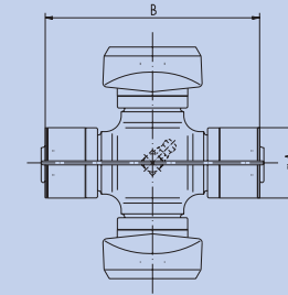
Gelenk Kreuz-Sätze für Half Round Yokes
