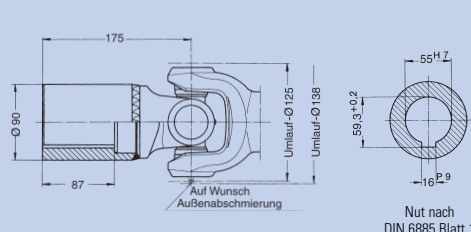
Beiderseits Anschlussnabe ohne Passfedern Endnummer: 0.113.XX2 mit Passfedern Endnummer: 0.113.XX3
