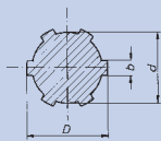
Keilwellen DIN ISO 14
