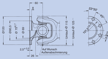
Normalflansch Endnummer: 0.112.XX0
