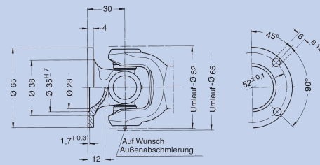
Größerer Flansch Endnummer: 0.105.XX1
