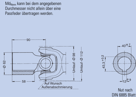
Anschlussnabe ohne Passfedernut Endnummer: 0.110.XX2 mit Passfedernut Endnummer: 0.110.XX3
