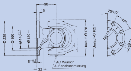
Größerer Flansch Endnummer: 0.120.XX1
