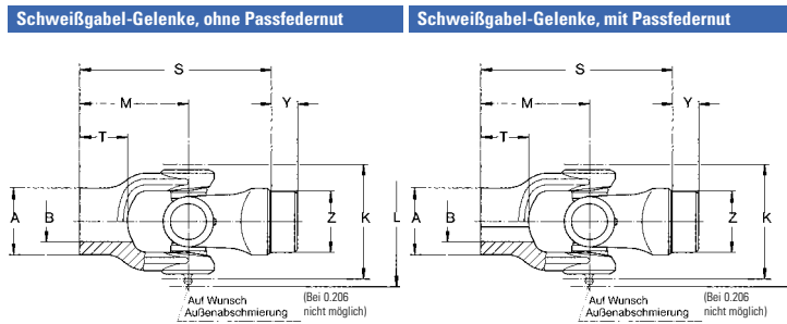
Passfedernut nach DIN 6885, Blatt 1
