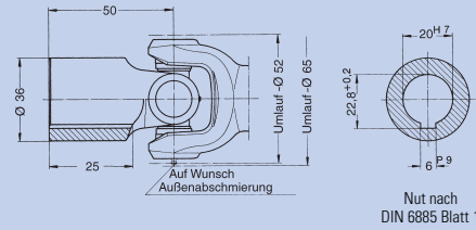
Beiderseits Anschlussnabe ohne Passfedernut Endnummer: 0.105.XX2 mit Passfedernut Endnummer: 0.105.XX3
