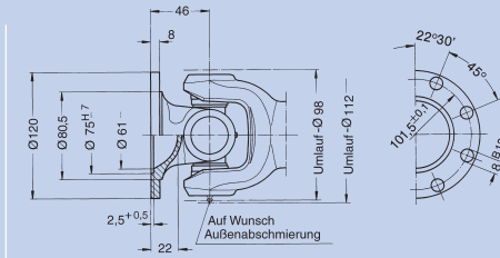
Beiderseits größerer Flansch Endnummer: 0.110.XX1
