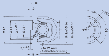
Größerer Flansch Endnummer: 0.107.XX1
