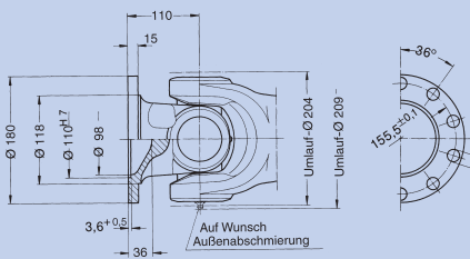
Normalfansch Endnummer: 0.122.XX0
