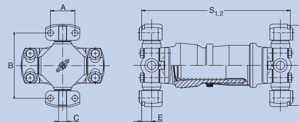
Bauform 130, Kurzausführung Endnummer: 0.9XX.130
