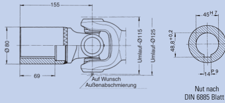
Beiderseits Anschlussnabe ohne Passfedern Endnummer: 0.112.XX2 mit Passfedern Endnummer: 0.112.XX3
