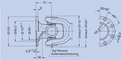
Beiderseits Flansch für größeren Beugungswinkel Endnummer: 0.112.XX5
