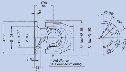
Größerer Flansch (Ø 165 mm) Endnummer: 0.117.XX1 Klammermaße sind gültig für Kurzausführung I
