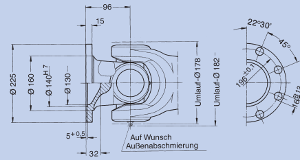
Beiderseits größerer Flansch Endnummer: 0.120.XX1
