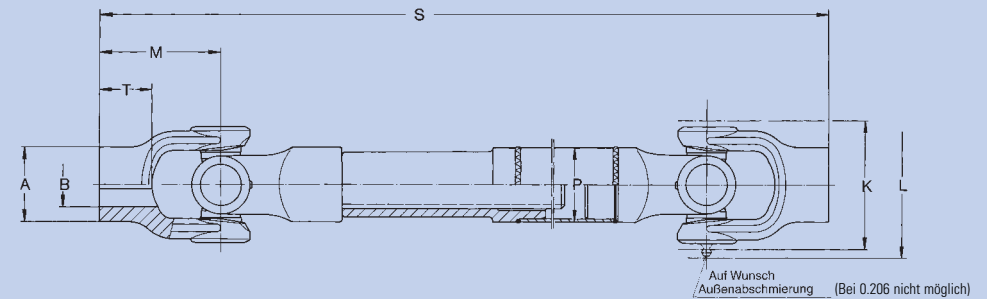
Beidseitig mit Passfedernut DIN 6885, Blatt 1; Endnummer: 0.204.XX3 Passfedernut nach DIN 6885, Blatt 1 Beidseitig mit Passfedernut DIN 6885, Blatt 1; Endnummer: 0.204.XX4
