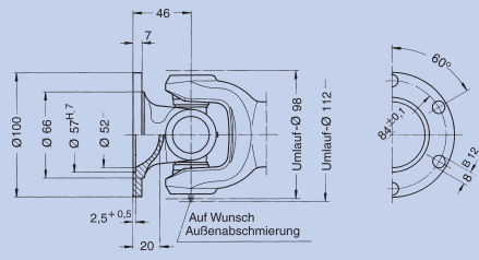
Normalflansch Endnummer: 0.110.XX0
