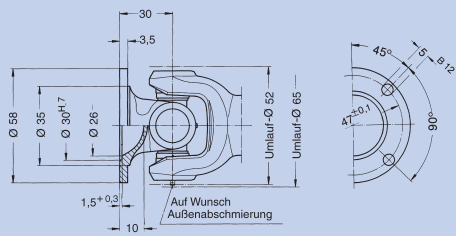
Normalflansch Endnummer: 0.105.XX0
