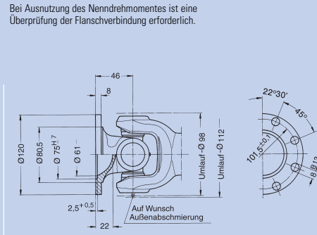
Größerer Flansch Endnummer: 0.110.XX1
