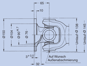
Beiderseits Normalflansch Endnummer: 0.148.XX0
